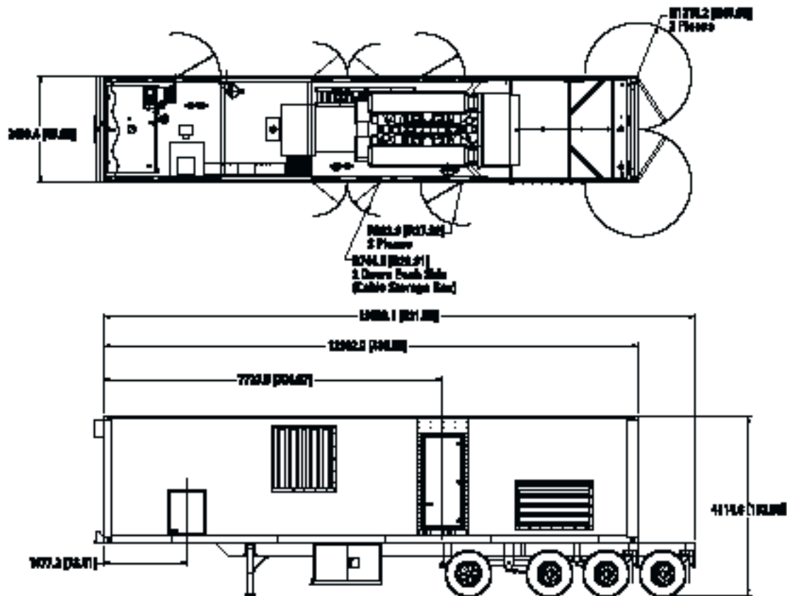
Container Dimensions
