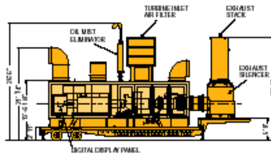
Generator Set Module
